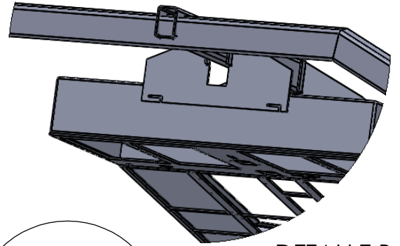
DETALLE B ESCALA 1 : 10
